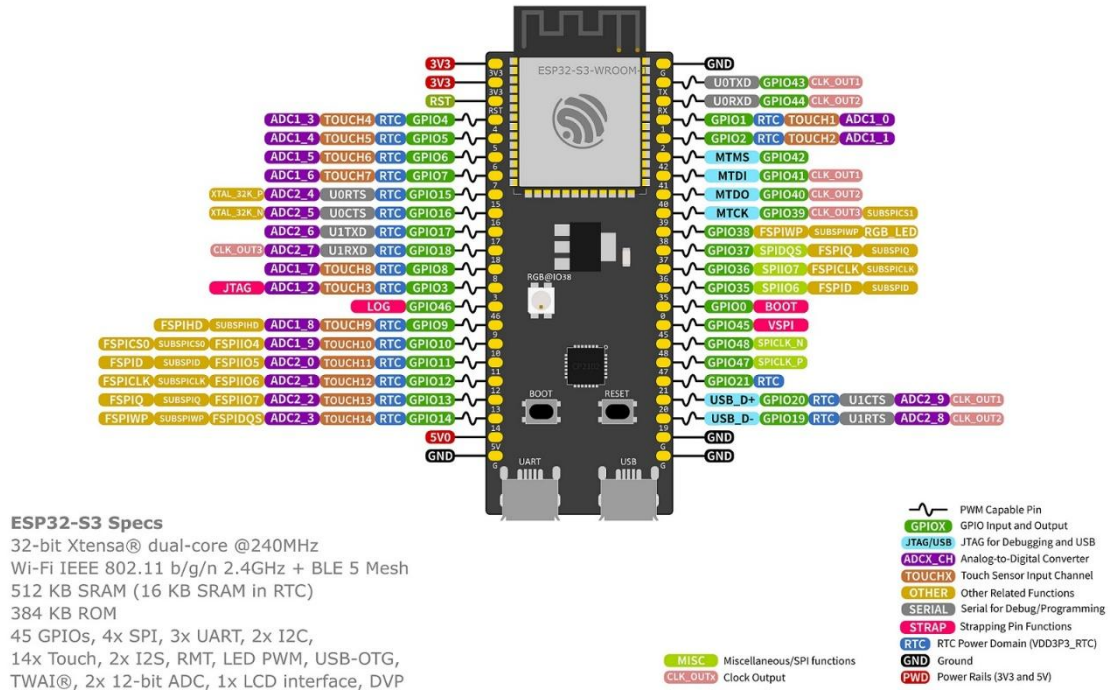
ESP32-S3-Module 管脚布局
